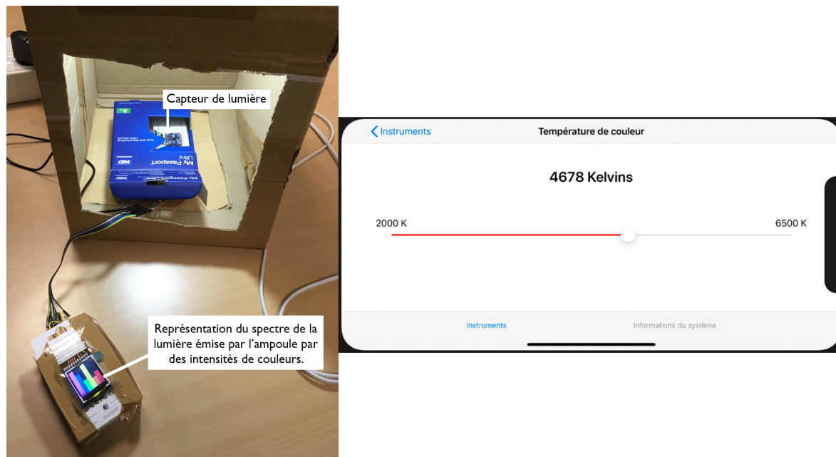
FIGURE 5.12 – Dispositif Teco. À gauche : Microcontrôleur Arduino permettant de capter la lumière émise par l'ampoule ; À droite : modification de la température de couleur de l'ampoule avec Lumière&Couleurs .
