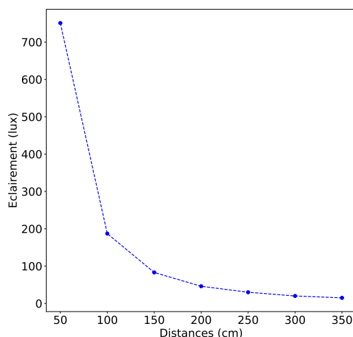
FIGURE 5.6 – Exemple de loi en carré inverse.
