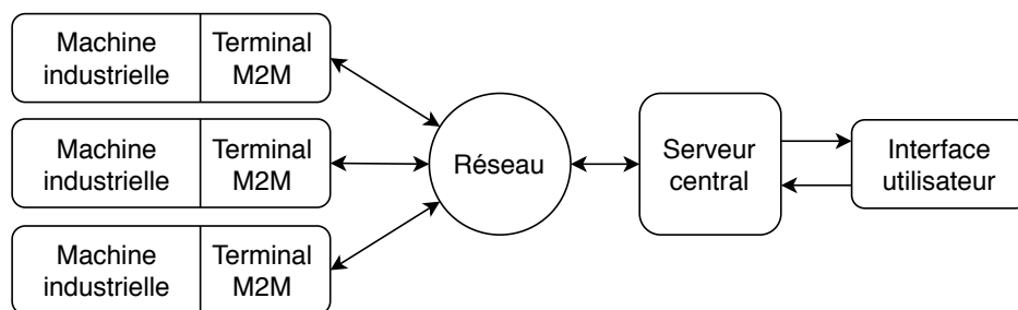
FIGURE 3.3 – Système Machine-to-Machine . Communication entre plusieurs machines (e.g. robot de ligne de montage, compteur électrique, distributeur automatique, véhicule) via un même réseau, centralisation dans un serveur de données métriques décrivant l'état des machines, visualisation des données et envoi de commandes depuis une interface utilisateur (Höller, 2014).
