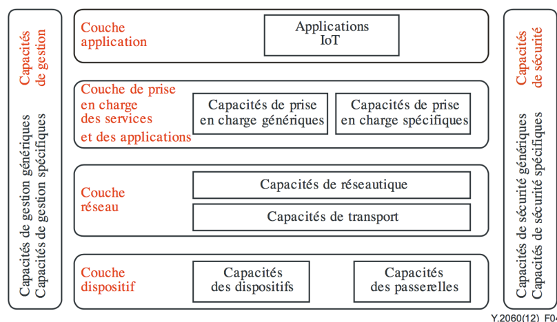
FIGURE 3.8 – Architecture de l'IdO selon l'UIT-T. Architecture de référence proposée par l'UIT-T dans sa Recommandation UIT-T Y.2060
