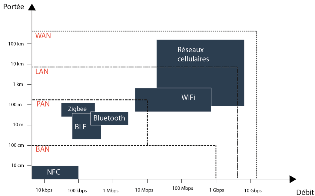
FIGURE 3.11 – Technologies de communication sans-fil selon la portée et le débit du signal (Roxin & Bouchereau, 2017b).
